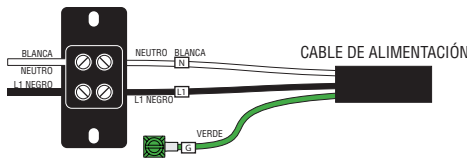
120VAC BIFILAR + TIERRA
